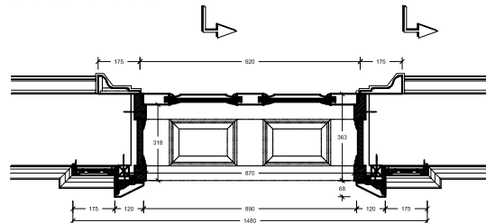
1:5 Plan Section A-A
