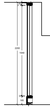
1:10 Height Section A-A
